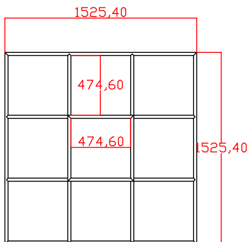
PLANTA BAIXA
