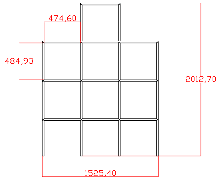
VISTA LATERAL
