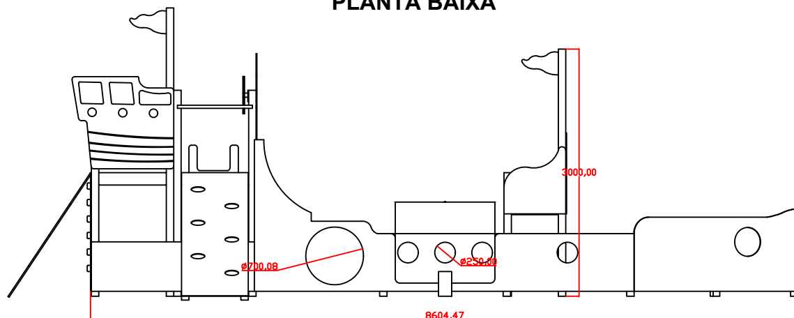
VISTA LATERAL
