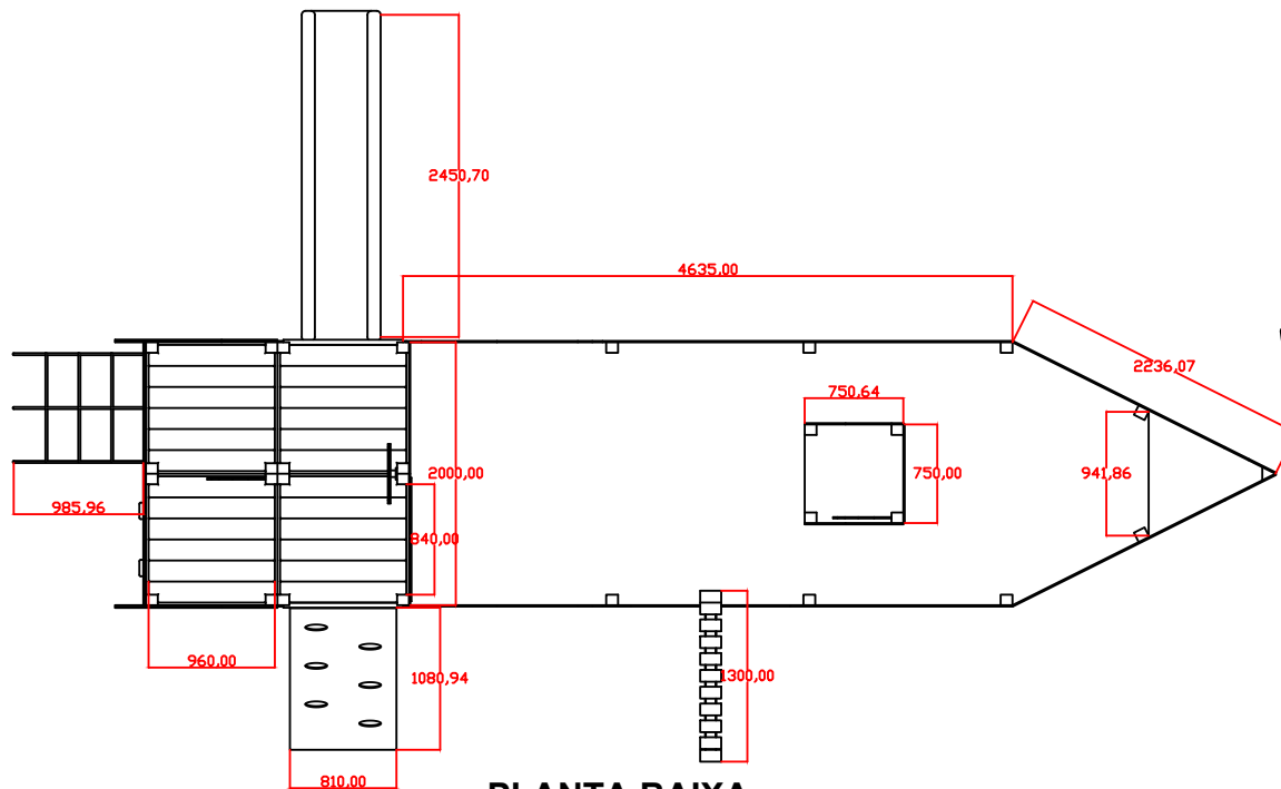
PLANTA BAIXA
